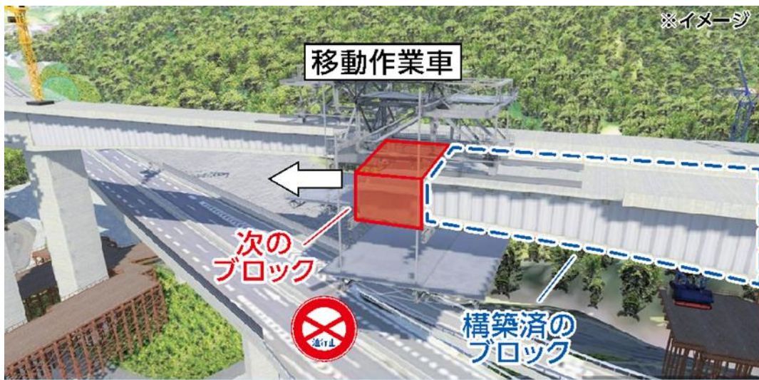
《移動作業車の移動(イメージ)》
