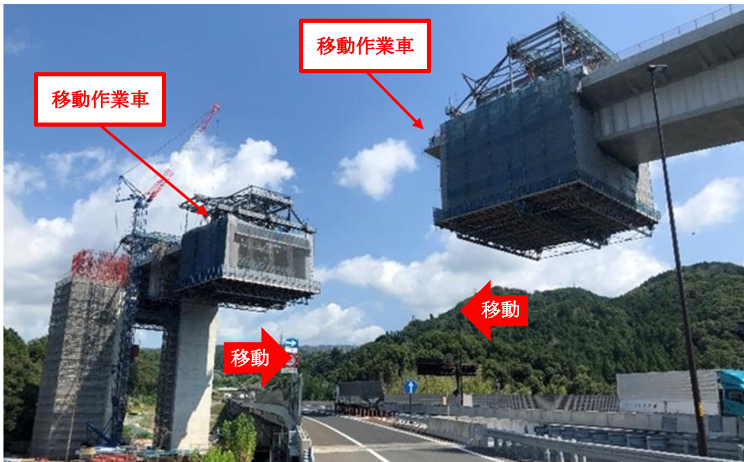
—橋梁上部工の架設工法—
