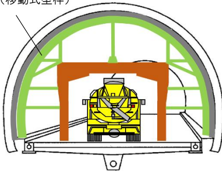
セントル(移動式型枠)
