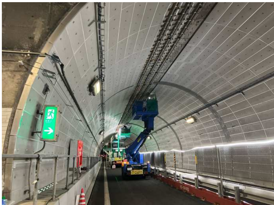
トンネル覆工内巻き工 施工状況
