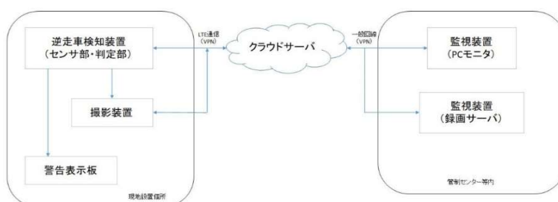
逆走検知システム概要図（クラウドサーバ使用時）
