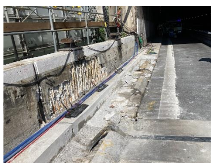
(武庫川橋壁高欄)
