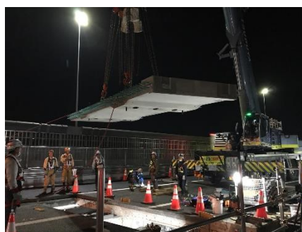
(新設床版架設)
