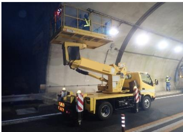
<トンネル照明内機交換作業>
