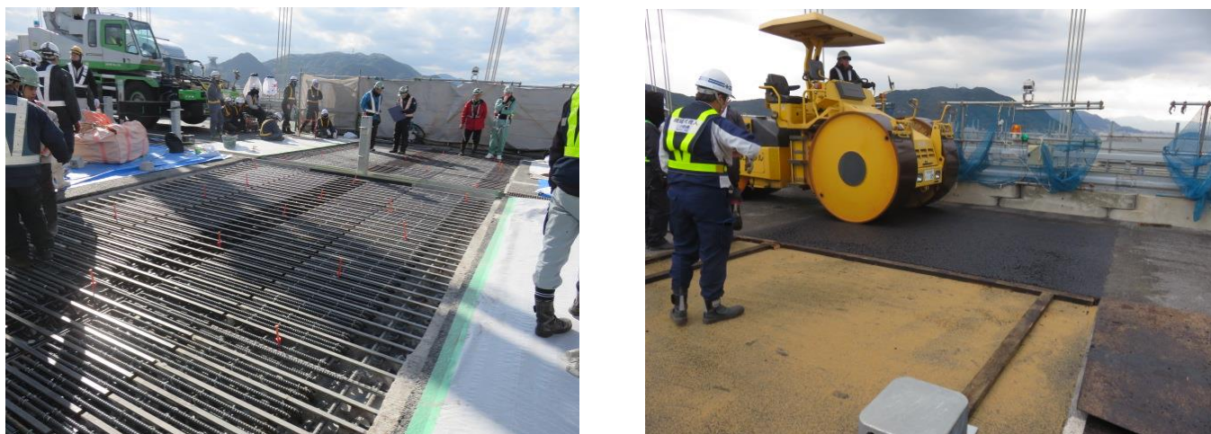
床版の設置、舗装状況
