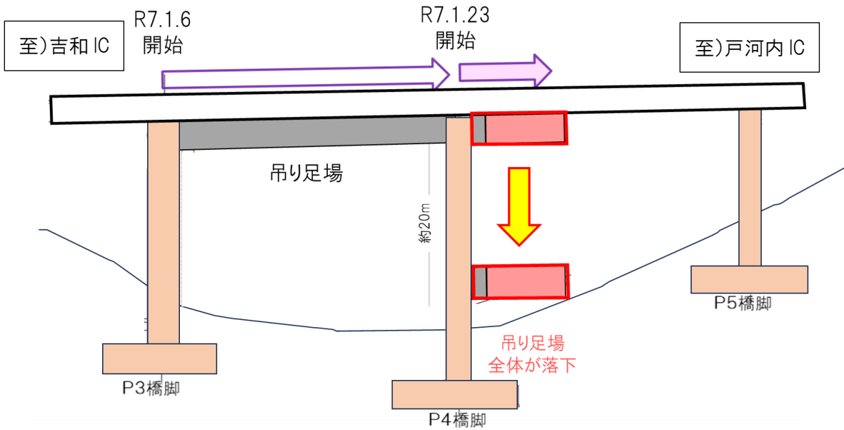
【縦断図】
