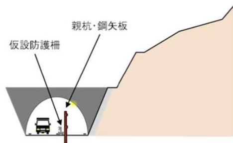
【高山トンネル下り線（東坑口）イメージ】 現在（1車線通行）
