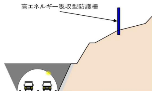
【高山トンネル下り線（東坑口）イメージ】 復旧対策後（2車線通行）
